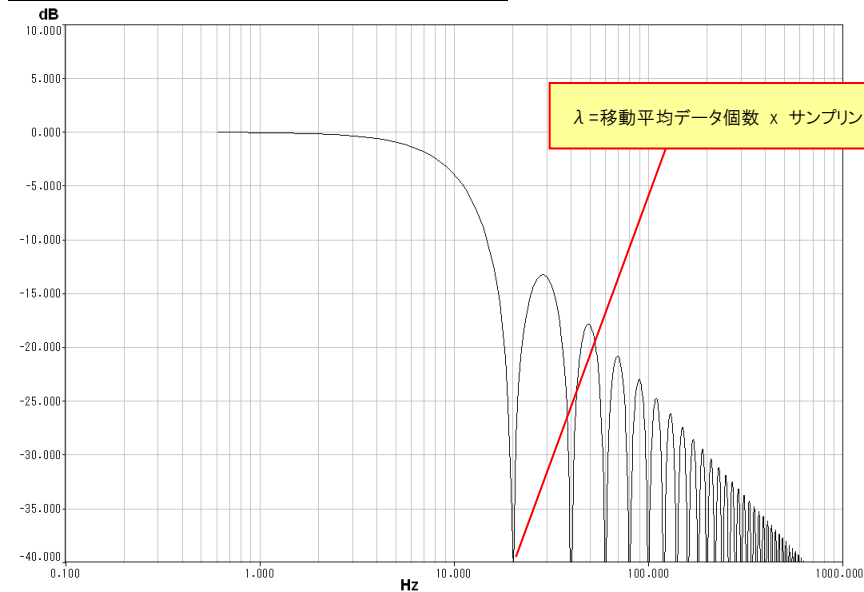
周波数軸上特性図(平均化個数を 20Hz 相当に設定時)
